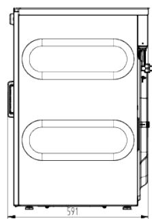
SC70 SEITENANSICHT
