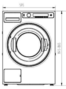
SC70 VORDERANSICHT
