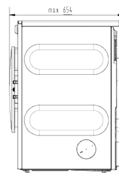
DAMV7 SEITENANSICHT
