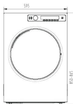
DAMV7 VORDERANSICHT
